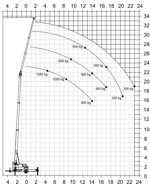
Diagram rozsahu plošiny
